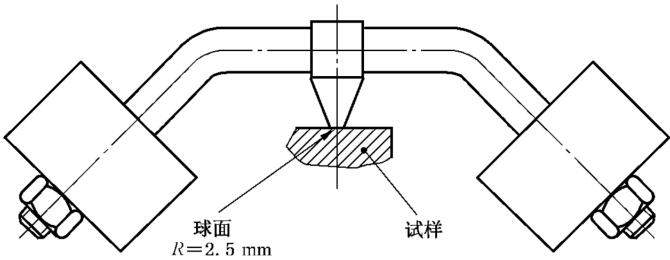
图 37 球压试验装置
