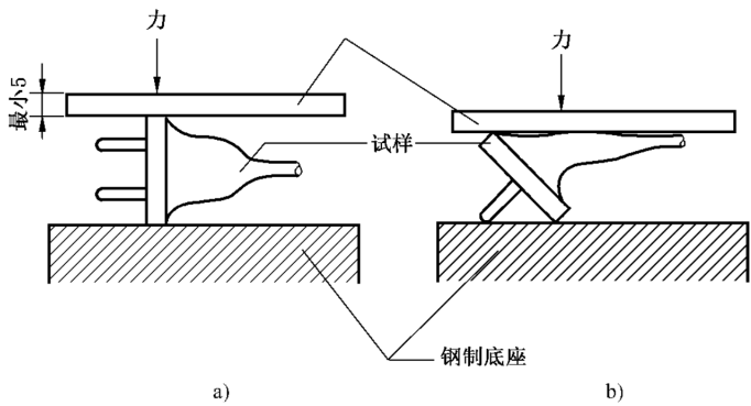
图 8 24.6 的压缩试验装置
