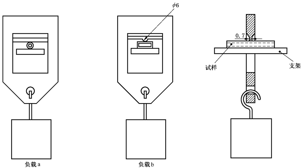
图 41 高温下压力试验装置
