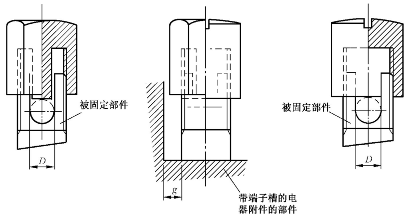
图 4 鞍型端子
