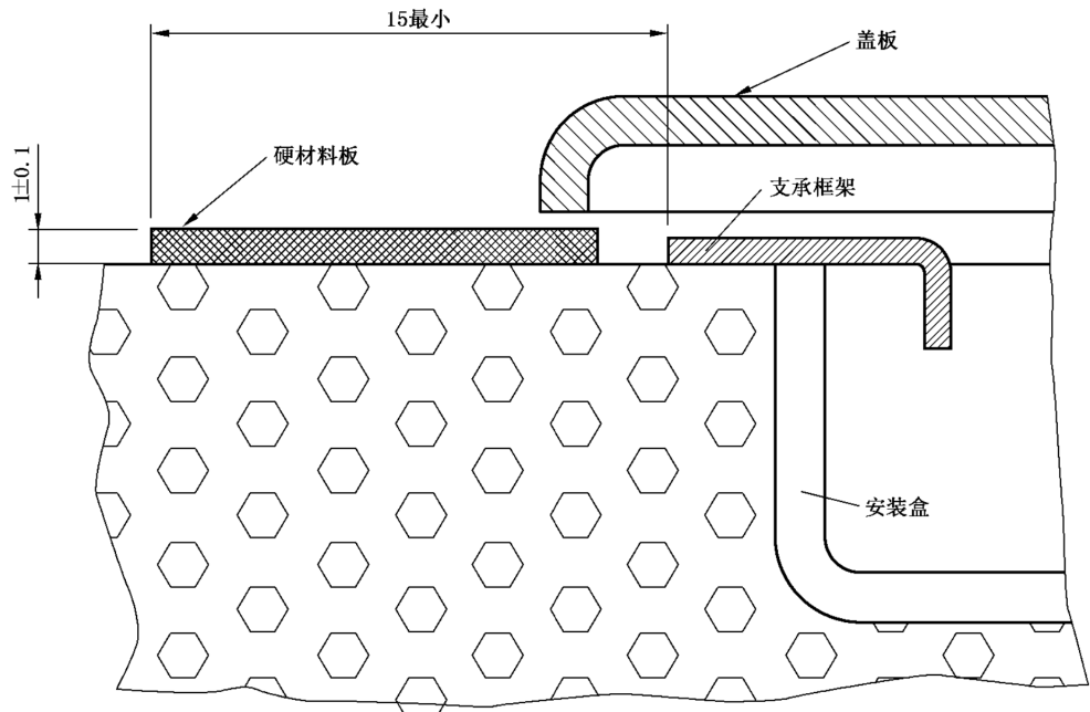
图 31 盖或盖板的试验装置
