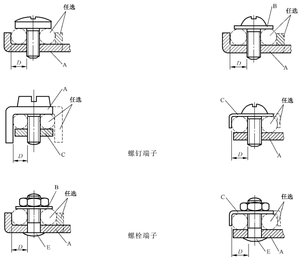
a) 不要求垫圈或夹紧板的螺钉/螺栓 b) 要求垫圈或夹紧板或防散部件的螺钉/螺栓
