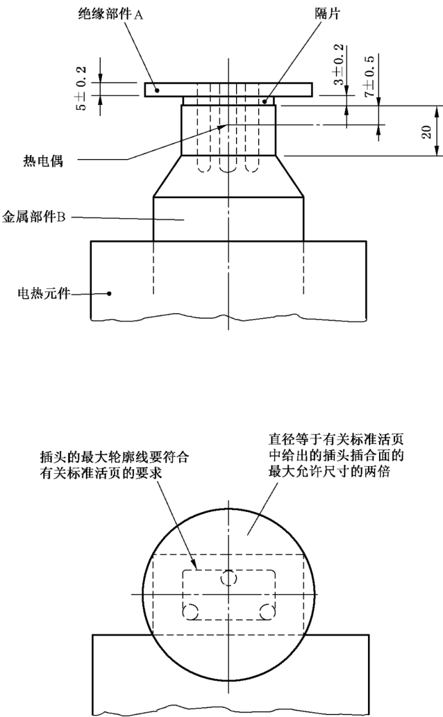
图 40 插头插销绝缘套耐非正常热试验装置
