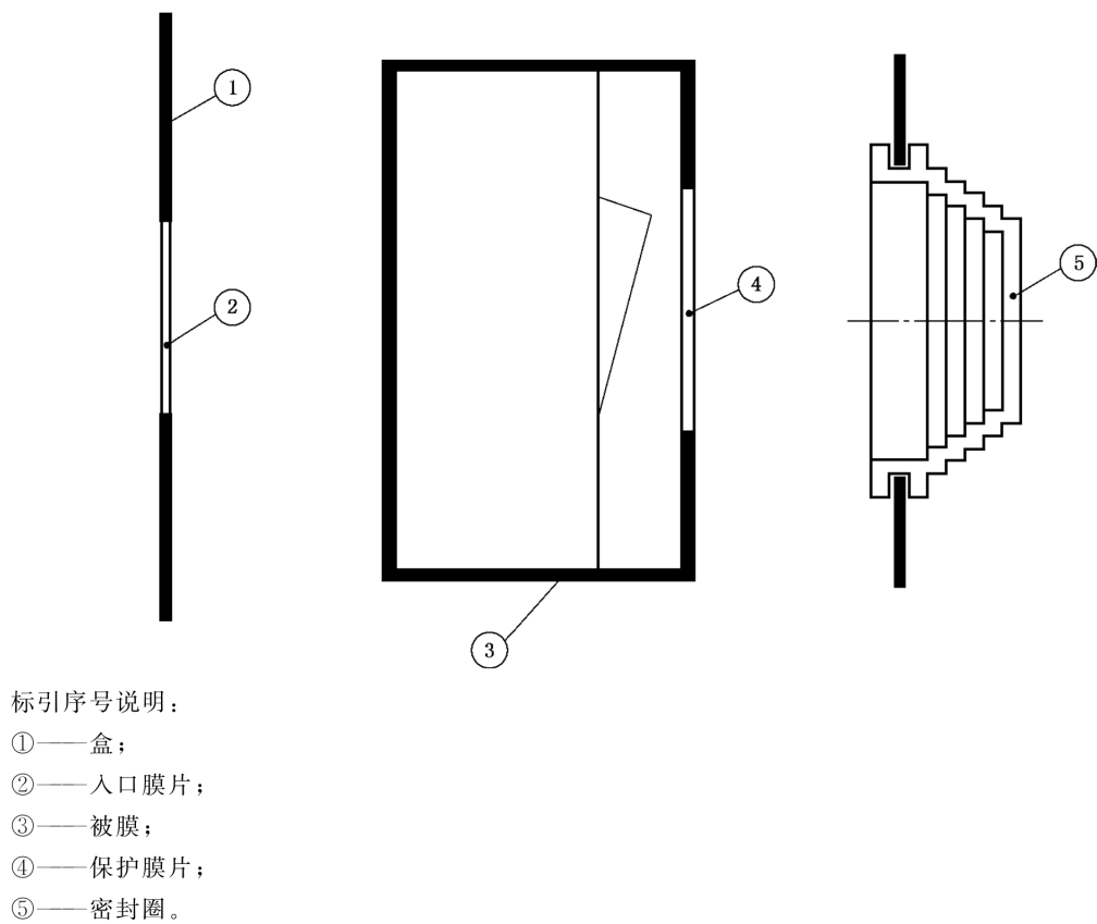
图 45 膜片与密封圈的示例图
