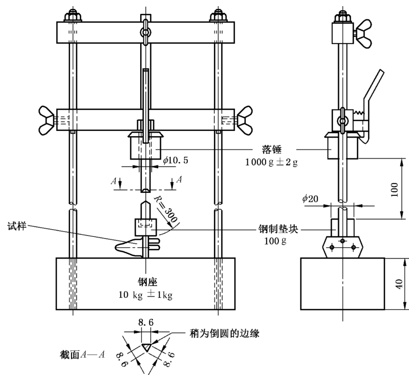
图 27 24.5 的低温冲击试验装置
